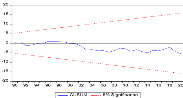
Fig. 1. CUSUM Test
